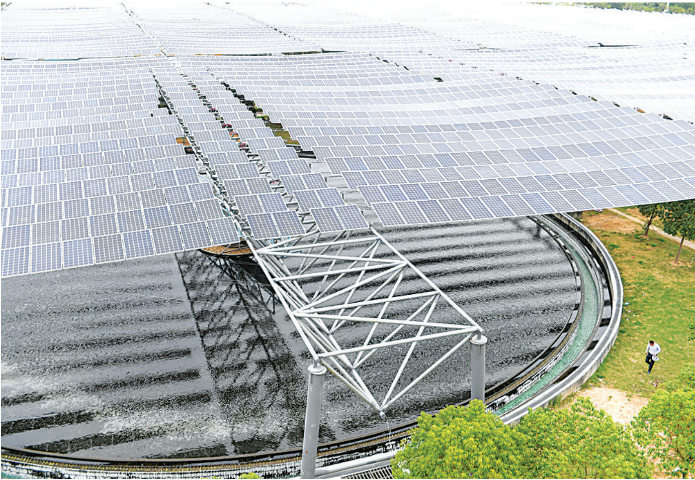
这是11月20日拍摄的福建省石狮市中心城区城市污水处理厂处理池上的分布式光伏发电项目。日前,位于福建省石狮市中心城区城市污水处理厂的3MW污水处理厂分布式光伏发电项目正式并网发电。这是当地首个高压并网光伏电站,总投资规模约2000万元,全站面积4000余平方米,总计安装10000块多晶硅太阳能电池板,一年预计可发电350万千瓦时。
