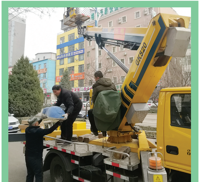
为了提高市区道路照明质量,保障市民夜间行车安全以及最大限度节约能源,12月10日,市区相关部门开始对凤山路存在问题的钠灯进行节能改造。据了解,通过改造换上新的LED灯具,具有更好的稳定性、舒适度、照明质量、使用寿命和节电效果。同时,也装饰了城市夜色,保障着夜归人的安全,有效解决市民夜间出行难和安全隐患问题。记者 郭炳中 摄
