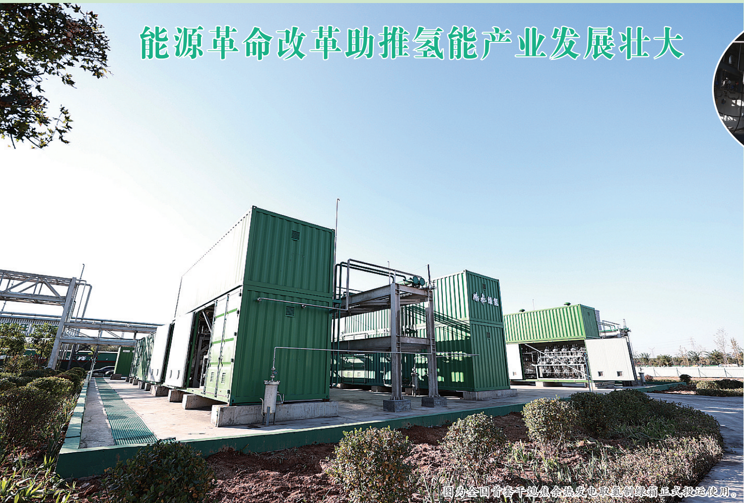
图为全国首套千吨级绿氢制备及储运制绿氨正式投运使用。
