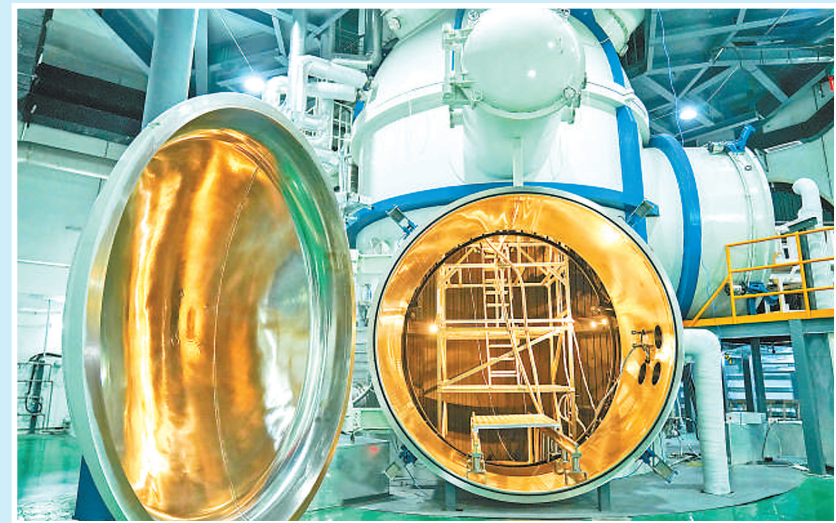
▲黑龙江哈尔滨新区科技创新城,我国航天领域首个大科学装置——空间环境地面模拟装置已进入试运行阶段,将用于探究空间环境对材料、器件、系统及生命体的影响规律和作用机制。 新华社记者 王松 摄
