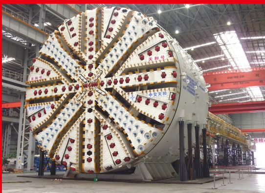
隧道掘进设备设计、制造、施工技术达到国际领先水平。“天和号”是中国研制的最大、直径达15.03米的泥水气压平衡复合式隧道掘进机。
